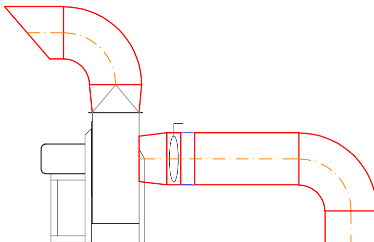
Ventilator GGE 802 18,5kW/1400RPM
