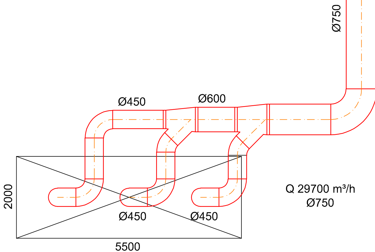
Ventilator GGE 802 18,5kW/1400RPM
